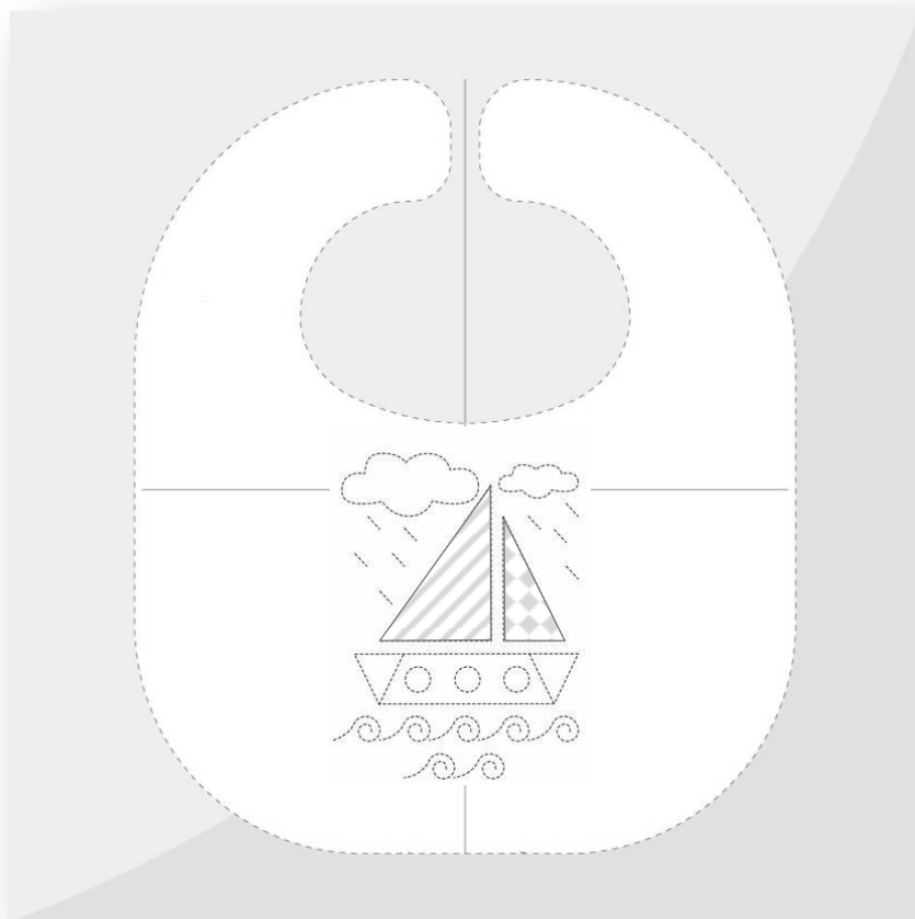
Рисунок 1 – Эскиз нагрудника
