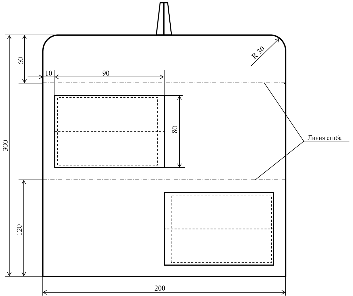
Рисунок 2 – Чертеж футляра
