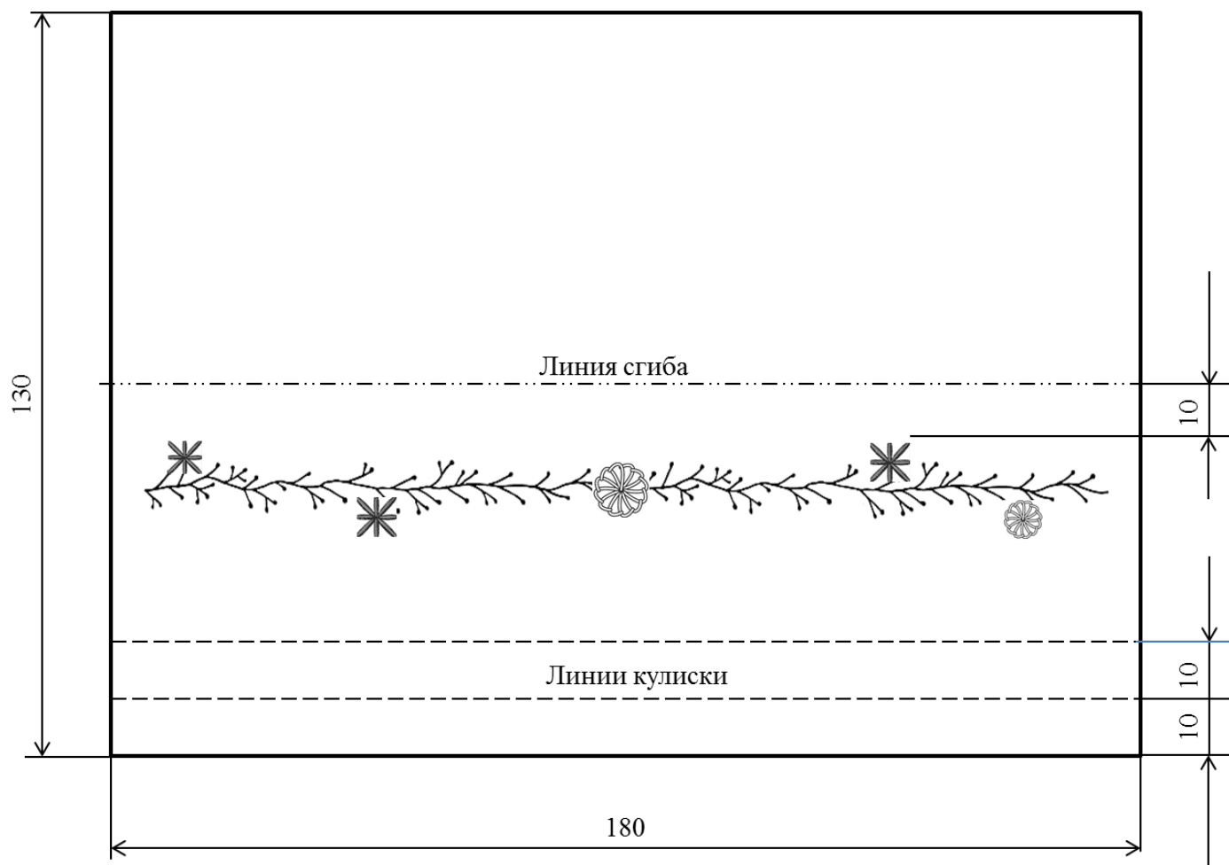
Рисунок 3 – Технический рисунок верхней части мешочка
