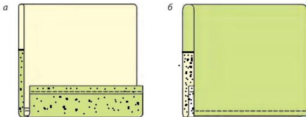
Рис. 2 . Складывание детали накладки перед обработкой боковых срезов: a — стачным швом; б — двойным швом
