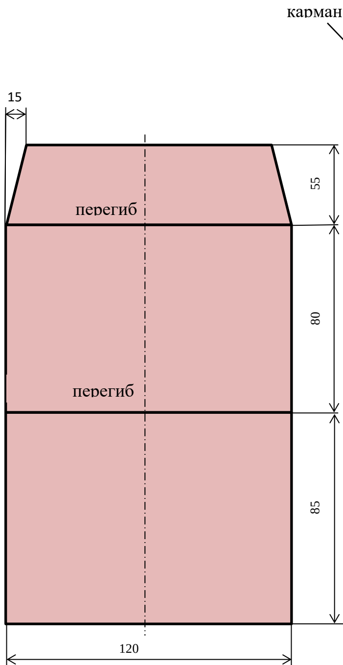
Рисунок 1- чертеж лекала деталей №1,2
